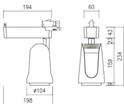
Technische Zeichnung
